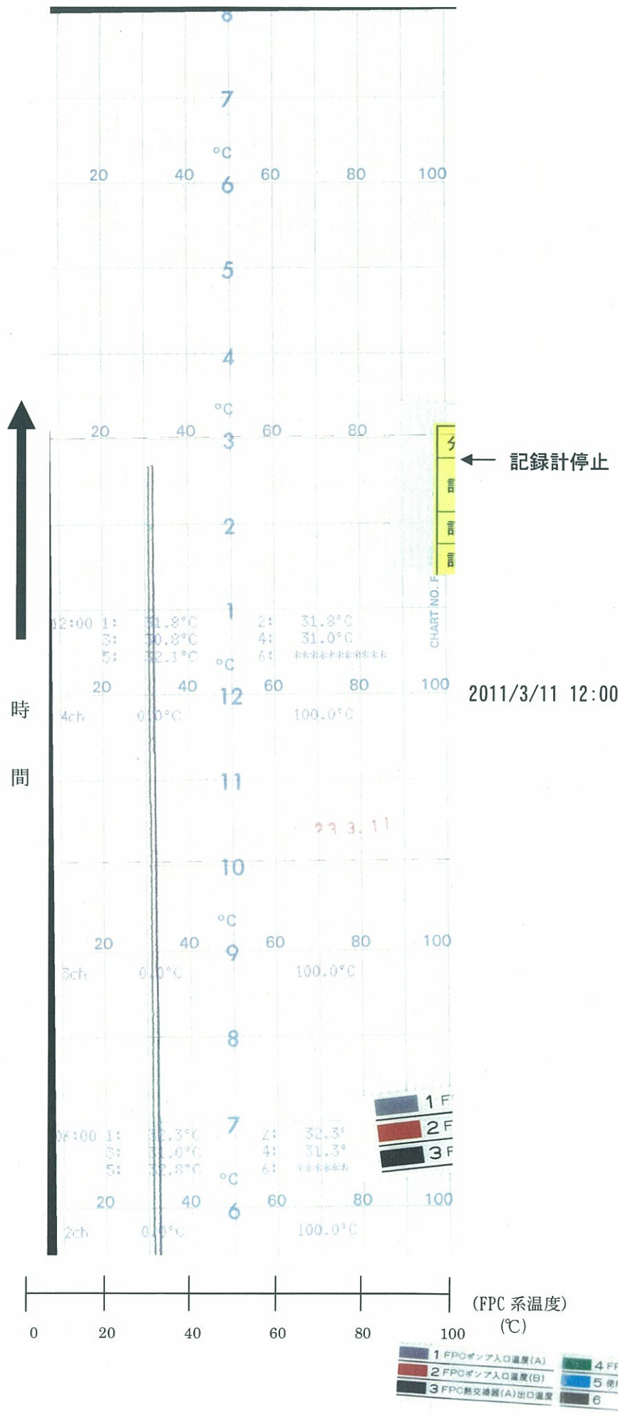
共用プール FPC系温度 (2/2)
