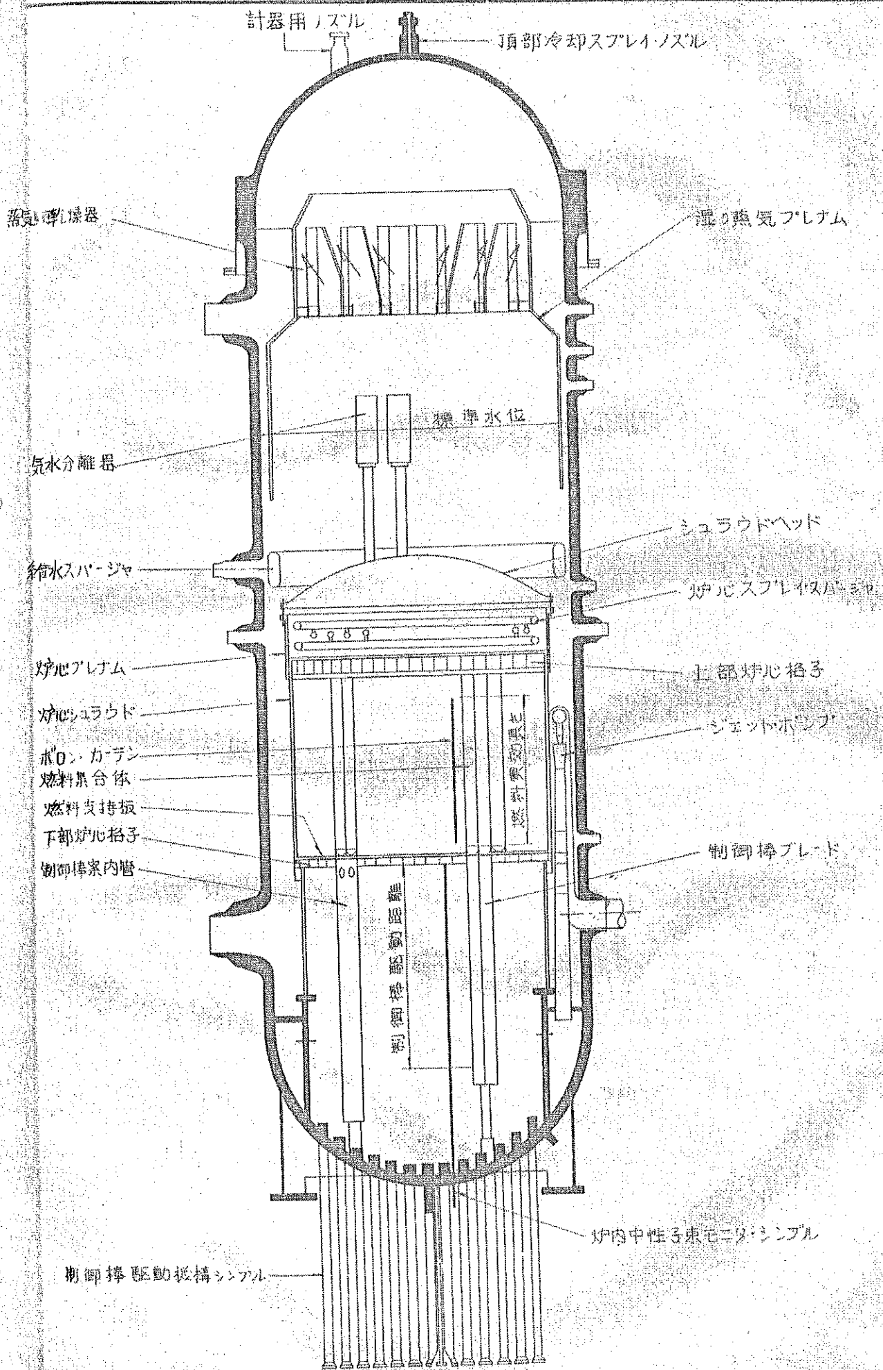
第 3.1-1 図 原子炉内部構造概略図
